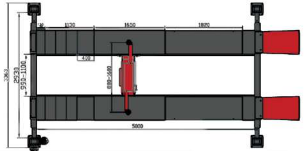
ابعاد الجهاز
