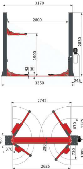
Line Draw ابعاد الجهاز
